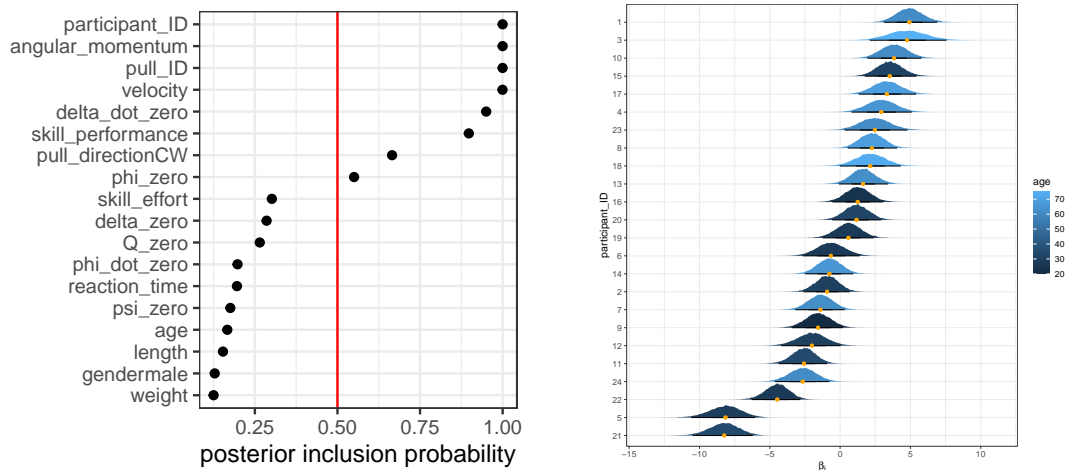
Figuur 4: Links: de aposterior kans dat een voorspeller in the verklarende model zit. Rechts: visualisatie van de vaardigheid van testpersoon om de fiets in evenwicht te houden.
