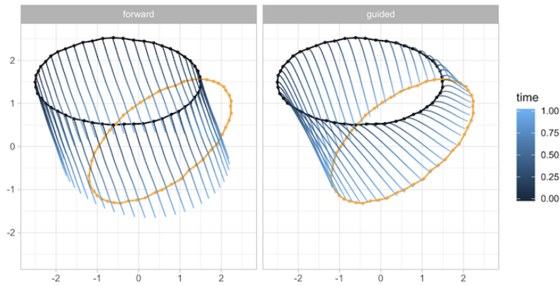
Figuur 15: Voorbeeld van een stochastisch model voor deformatie van vormen. Links: een realisatie van het voorwaardse model. Rechts: een realisatie van een proces dat de vormen interpoleert.
