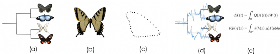
Figuur 14: (a) Fylogentische boom voor evolutie van vlinders. (c) toont landmark van de linker-voorvleugel van de vlinder in (b). (d): visualisatie van de statistische methode: een stochastisch model voor de verandering van de landmarks op de linkervoorvleugel. (e): stochastische differentiaalvergelijking voor het proces van de landmarks. Figuur gemaakt door Sofia Stroustrup.
